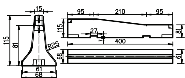
TLR3 (Reiff 2000 BSWF UE 115-81) אלמנט מעבר מגובה 115+81 ס"מ
