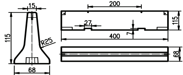
TLR3 (Reiff 2000 BSWF UE 115-81) אלמנט מעבר מגובה 115+81 ס"מ
