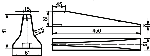
TLR4 (Reiff 2000 BSWF AE 81D) יחידת קצה מגובה 81+8 ס"מ
