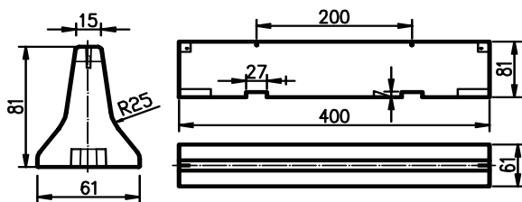
TLR1 (Reiff 2000 BSWF SE 81D) מעקות בטיחות ניידים לרמה T3
