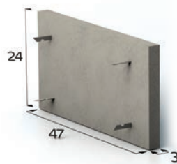
אופק אינטגרלי עוגנים במצב פתוח
