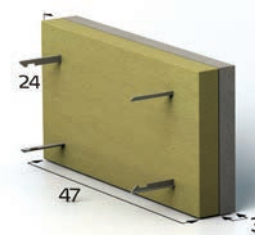
אופק אינטגרלי T לבידוד תרמי עוגנים במצב פתוח
