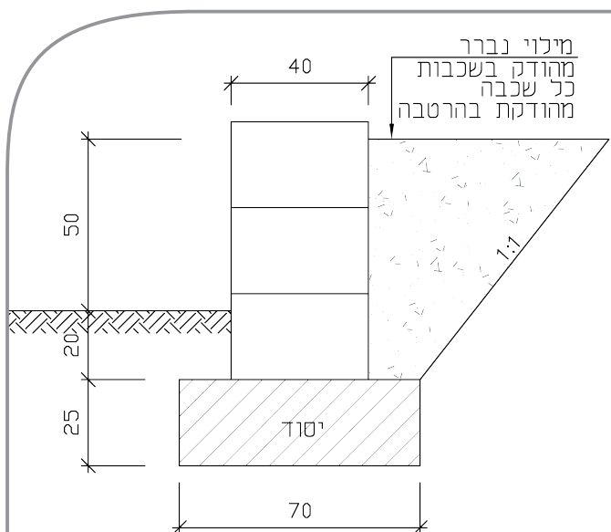
חתך אופייני
