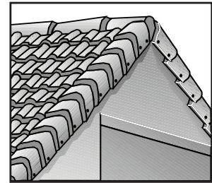
רעף צד דגם דרום אפריקה
