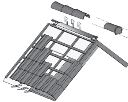
עקרון פעולה גג מאוורר
