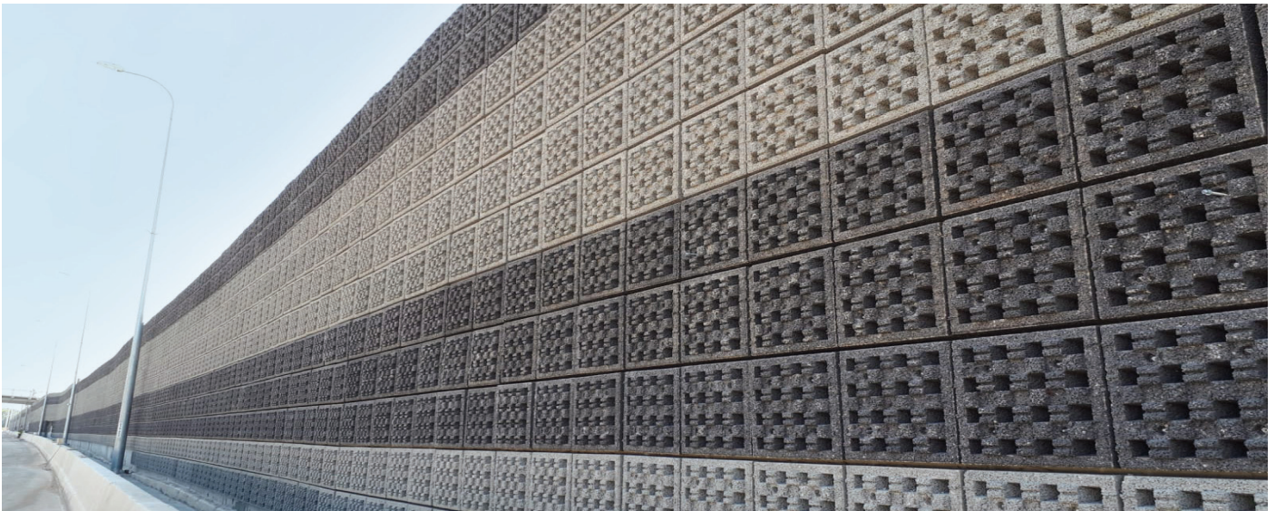
קיר אקוסטי "סונופור" דרך 531/20 הרצליה. יינן מהנדסים.
