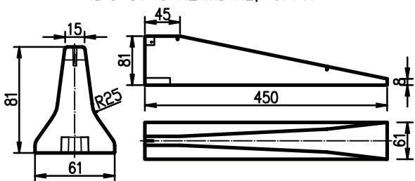
TLR4 (Reiff 2000 BSWF AE 81D) יחידת קצה מגובה 8+81 ס"מ
