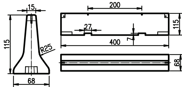
TLR2 (Reiff 2000 BSWF SE 115D) מעקות בטיחות קבועים לרמה H2
