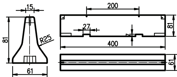
TLR1 (Reiff 2000 BSWF SE 81D) מעקות בטיחות ניידים לרמה T3
