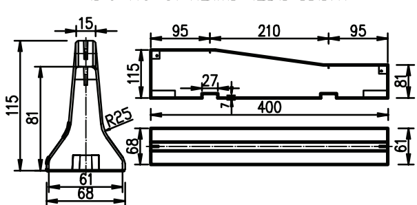
TLR3 (Reiff 2000 BSWF UE 115-81) אלמנט מעבר מגובה 115+81 ס"מ
