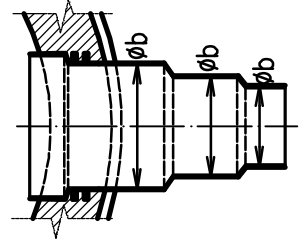
פרט יציאה אוניברסלית
