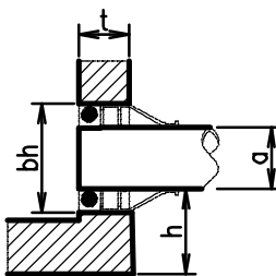
כניסה/יציאה אקרבייס דגם B
